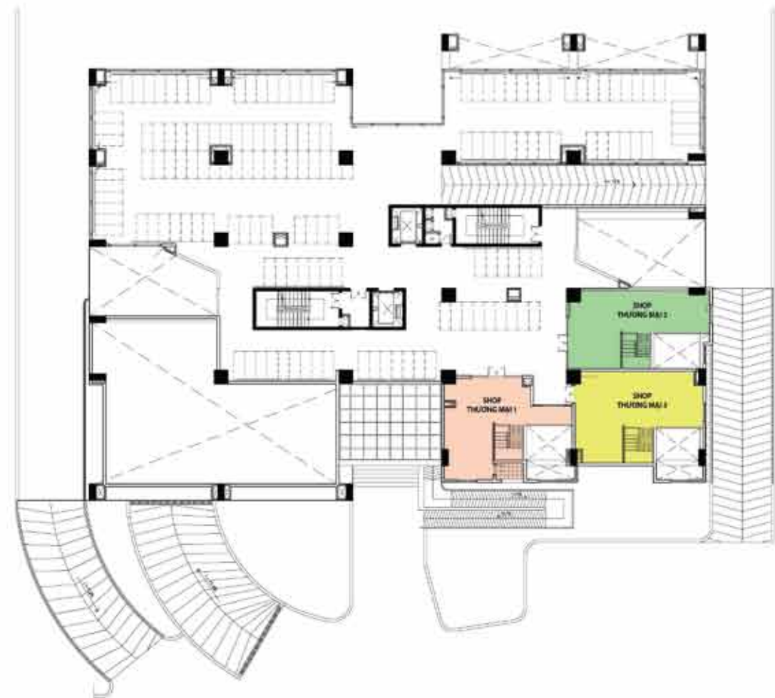
MẶT BẰNG SHOP THƯƠNG MẠI TẦNG LỬNG
